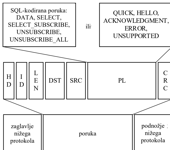
Slika 3.3. Oblićje i ućahurivanje poruka metaprotokola
