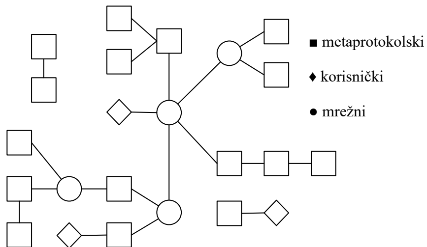
Slika 3.1. Primjer arhitekture
