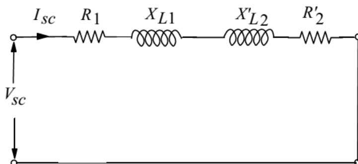
Slika 3-5. Nadomjesna shema pokusa kratkog spoja transformatora
