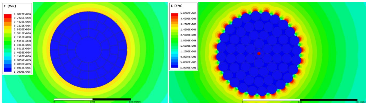
Slika 7.10: Prikaz raspodjele el. polja na vodiču (lijevo – ACCC, desno ACSR vodič)
