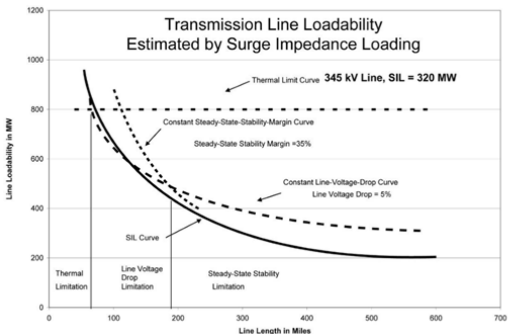
Slika 5.6: Ograničenja prijenosa snage na dalekovodu [14]
