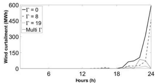
Fig. 3. Wind curtailment.
