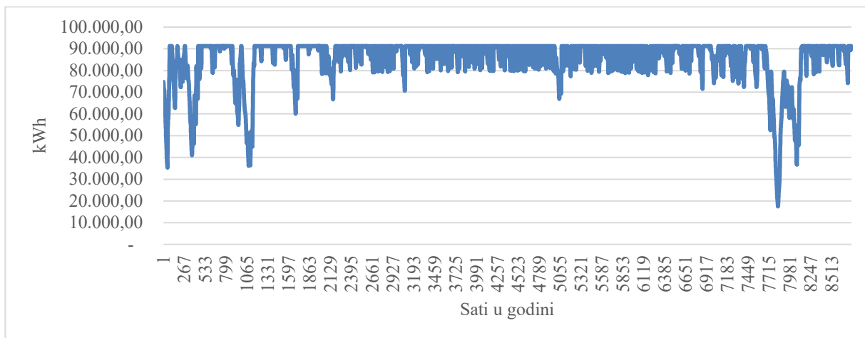
Slika 7.21: Dinamika spremnika tijekom 6. simulirane godine
