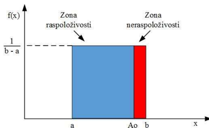
Slika 6.12: Korištena uniformna razdioba za Monte Carlo simulaciju
