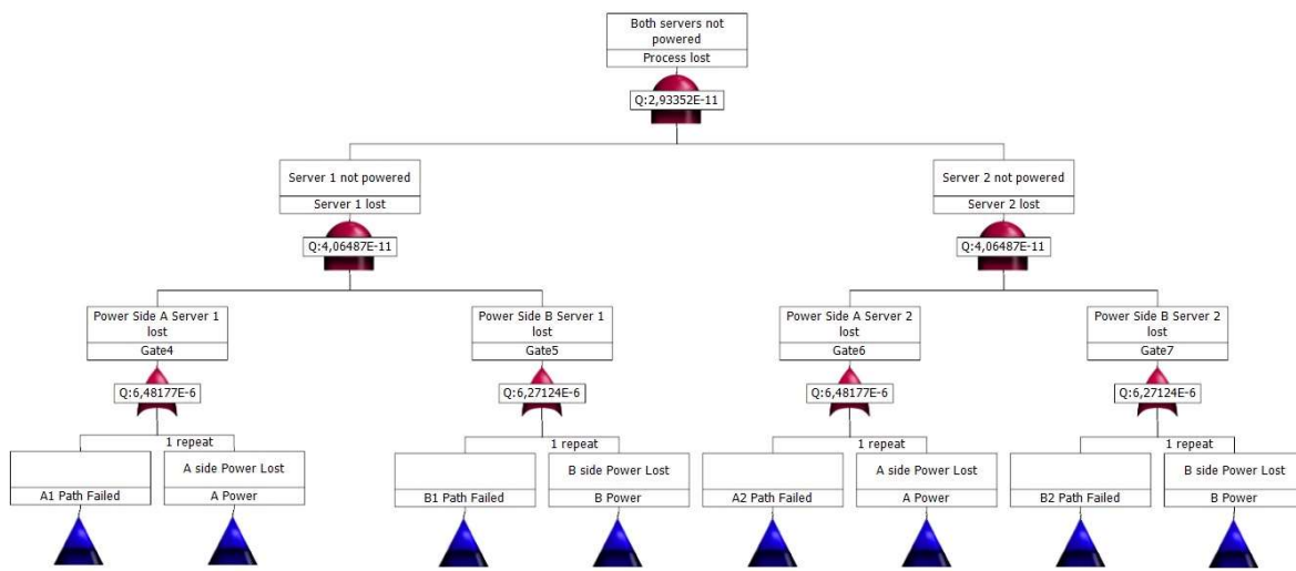
Slika 6.6: DFTA za cijelu arhitekturu [9]
