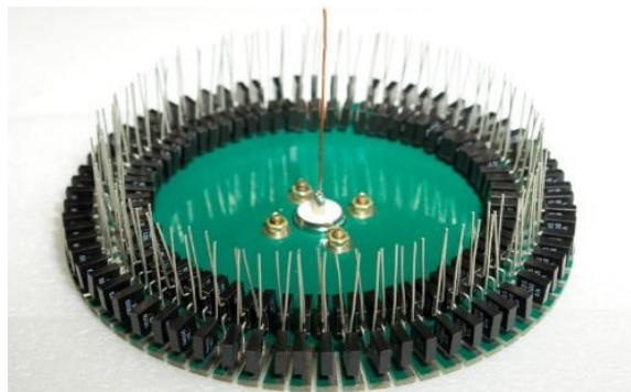
Slika 2.3 Dva reda Vishay otpornika na jednom od diskova shunta nazivne struje 10 A
