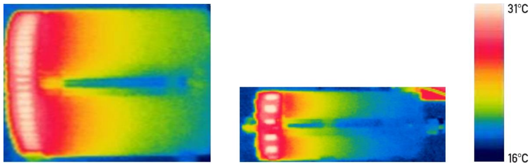
Slika 3.3 Temperaturna distribucija pri nazivnoj struji fotografirana termičkom kamerom (za shunt 5 A i 100 mA)
