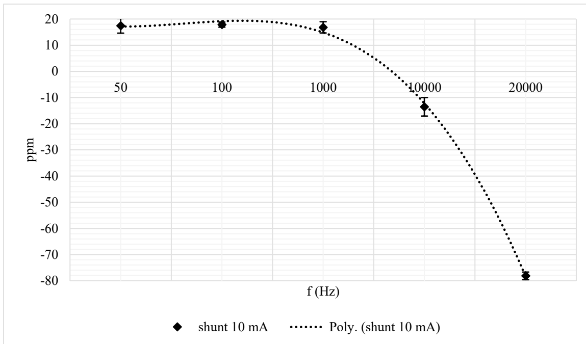
Slika 3.29 ac-dc razlika za shunt od 10 mA na frekvencijskom opsegu 50 Hz – 20 kHz [68]
