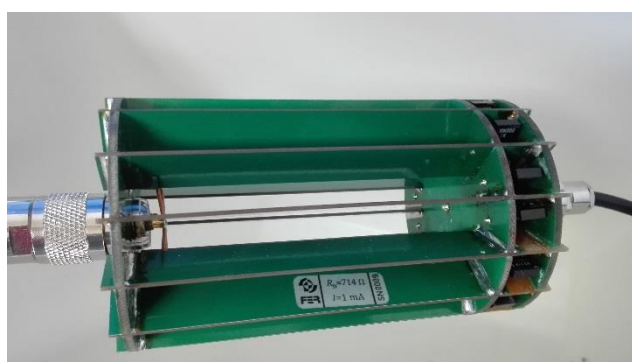
Slika 3.8 Mjereni strujni shunt unutar zračne komore
