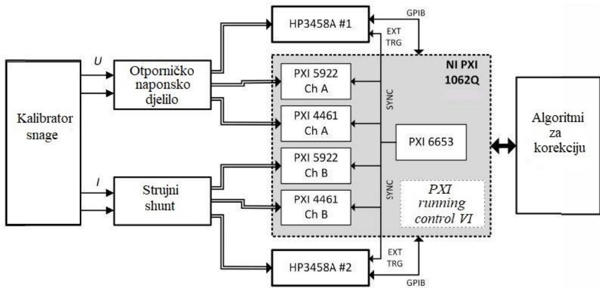
Slika 5.4 Shema mjernog sustava [106]
