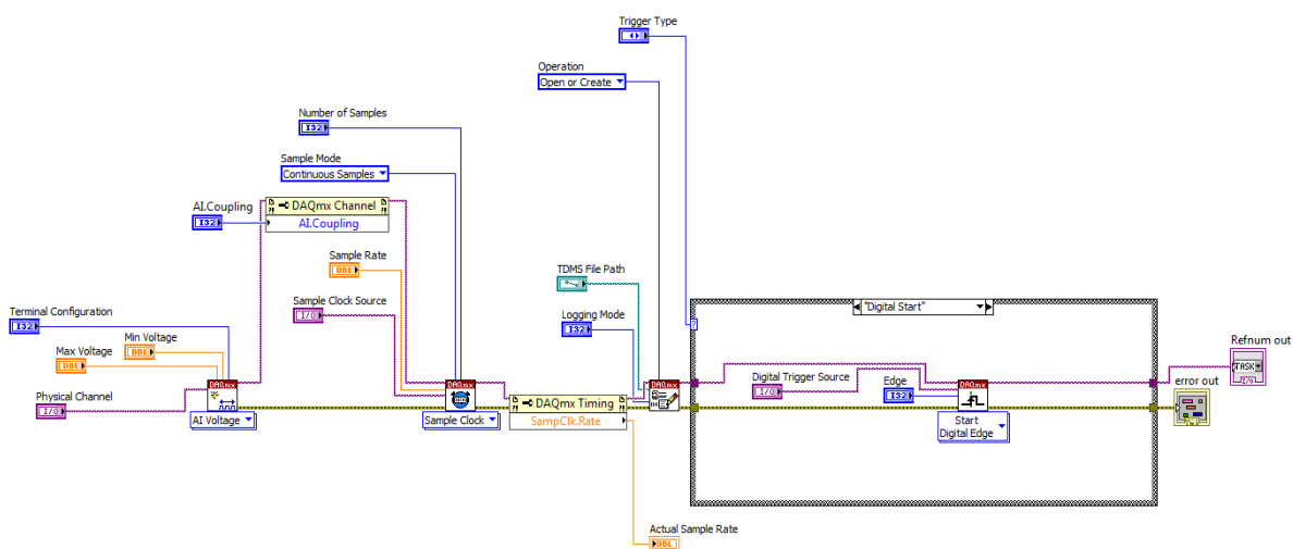
Slika 6.5 Potprogram za konfiguraciju mjerne kartice NI 4461
