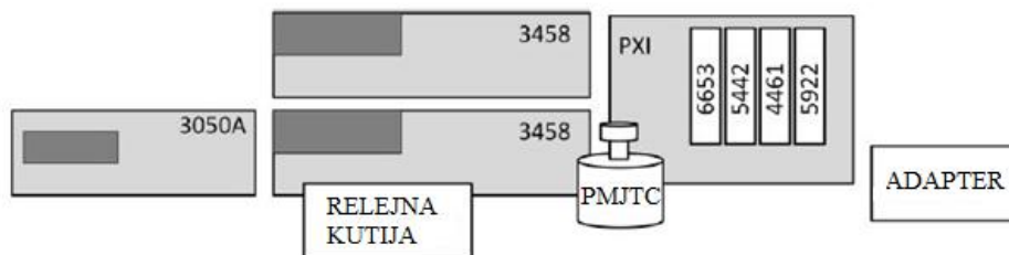
Slika 4.2 Mjerna oprema uz simbolički prikaz
