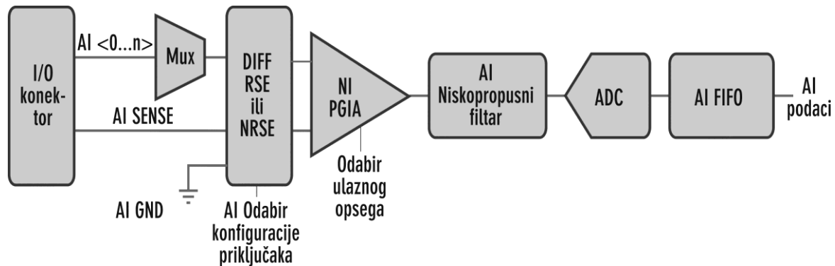
Slika 2.6 Sklopovske komponente DAQ uređaja
