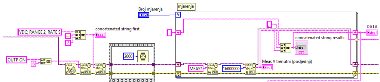
Slika 6.1 Dio programa za mjerenje napona digitalnim multimetrom (RIGOL DM3061) prilikom mjerenja TCR-a
