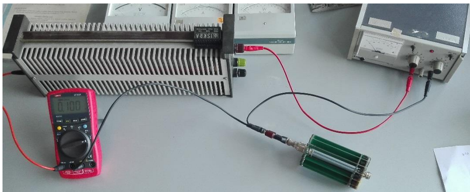
Slika 3.1 Mjerni strujni krug za praćenje temperaturne distribucije pomoću termičke kamere (za shuntove sa 14 rebara)
