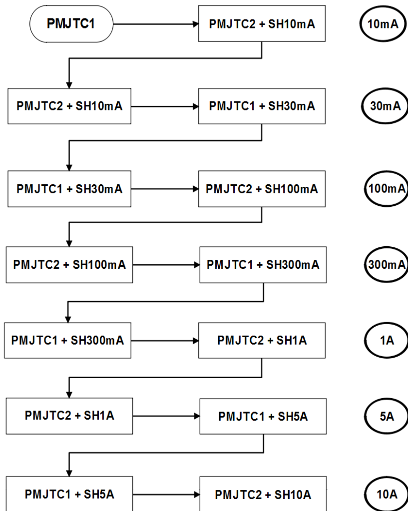
Slika 3.25 Step-up procedura za mjerenje ac-dc razlike (prikazano do koraka u kojem je nazivna struja od 10A) [68]
