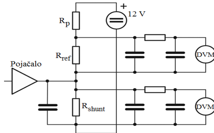
Slika 3.14 Shema mjernog električnog kruga za određivanje PCR-a strujnih shuntova [31]
