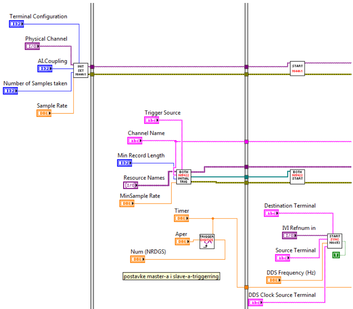
Slika 6.4 Dio glavnog programa za usporedbu mjernih instrumenata u sklopu digitalnoga vatmetra (radi jednostavnosti je prikazan samo dio glavnog programa bez detaljnog uvida u potprograme (tzv. subVIs ))
