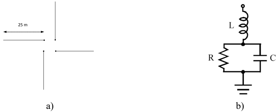
Slika 6.6: Konfiguracija uzemljivača stupa 4 x L (a) i nadomjesni model uzemljivača stupa (b)
