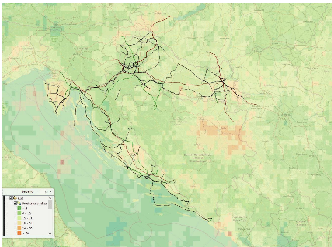
Slika 3.8: Gustoća atmosferskih pražnjenja oblak-zemlja u 2018. godini
