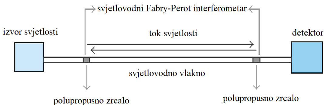
Slika 1.9: Prikaz osnovnih elemenata Fabry-Perot interferometarskog sustava [2].
