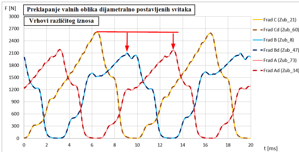
Slika 8.2 Svojevrsna razlika valnih oblika sile u slučaju nesimetričnog električnog opterećenja uz poklapanje valnih oblika dijametralno postavljenih svitaka
