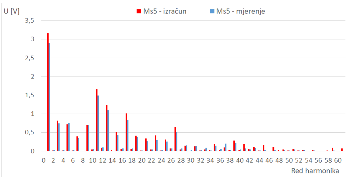
Slika 7.20 Usporedba harmonijskog sastava napona induciranog u mjernom svitku Ms5 određenog MKE proračunom i mjerenjem za nesimetrično opterećenje U=400\text{ V} , S=104\text{ kVA} , \cos\varphi=1
