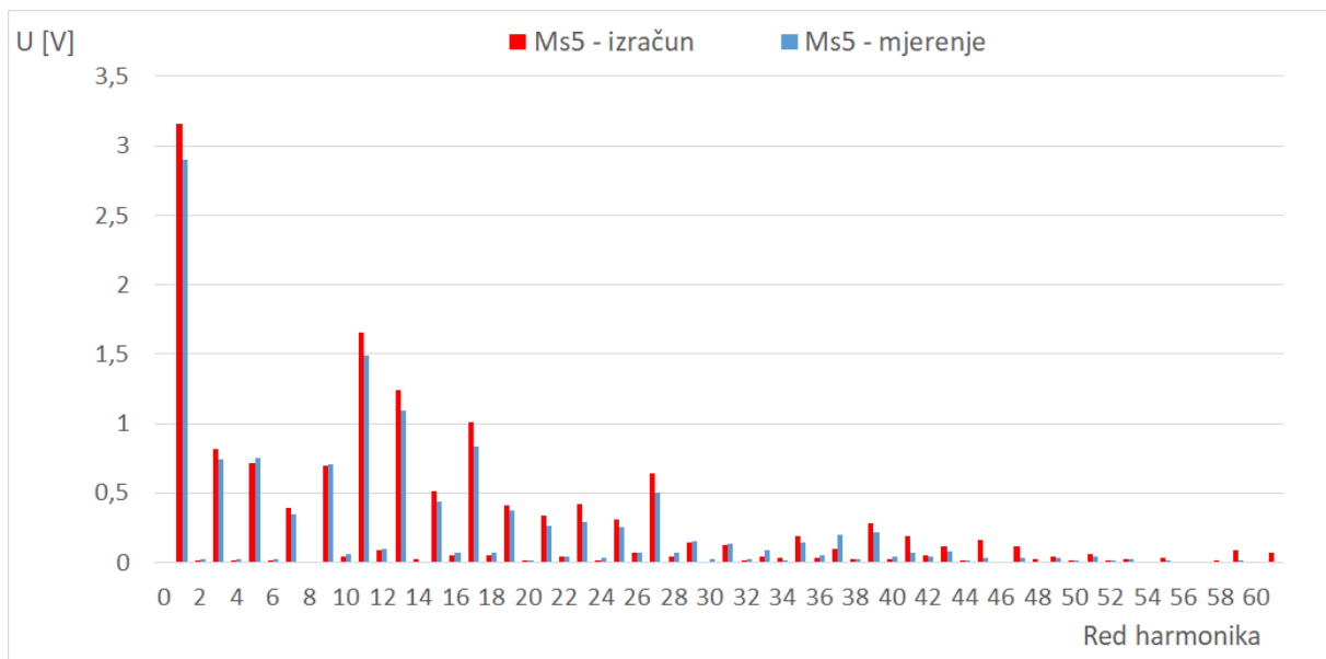
Slika 7.20 Usporedba harmonijskog sastava napona inducirano u mjernom svitku Ms5 određenog MKE proračunom i mjerenjem za nesimetrično opterećenje U=400 V, S=104 kVA, \cos\varphi=1
