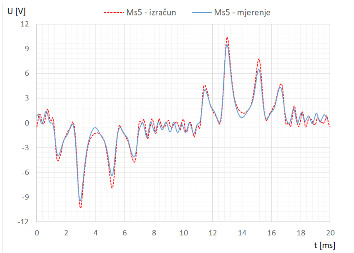
Slika 7.19 Usporedba valnog oblika napona inducirano u mjernom svitku Ms5 određenog MKE proračunom i mjerenjem za nesimetrično opterećenje U=400 V, S=104 kVA, \cos\varphi=1
