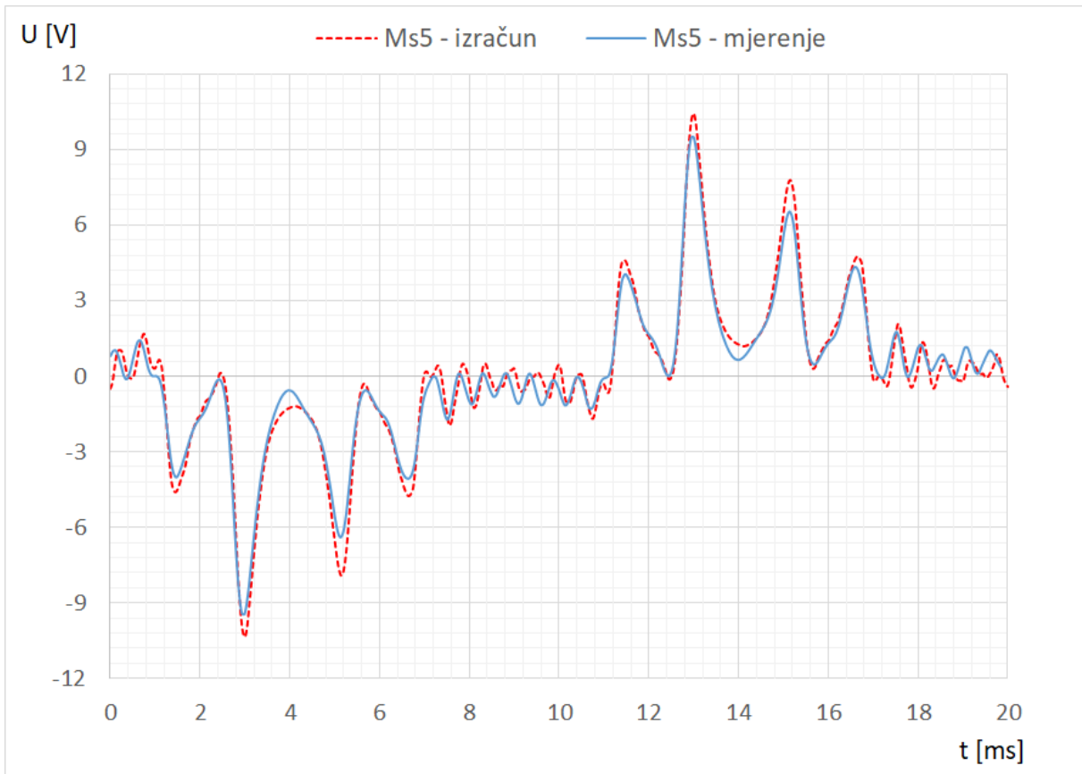
Slika 7.19 Usporedba valnog oblika napona induciranog u mjernom svitku Ms5 određenog MKE proračunom i mjerenjem za nesimetrično opterećenje U=400\text{ V} , S=104\text{ kVA} , \cos\varphi=1
