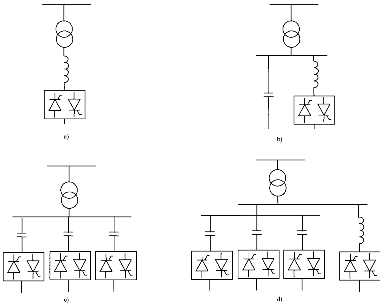
Slika 60: SVC konfiguracije: a) tiristorski upravljana prigušnica; b) tiristorski upravljana prigušnica s fiksnim kondenzatorom; c) tiristorski uklopiv kondenzator; d) tiristorski upravljana prigušnica s tiristorski uklopivim kondenzatorom
