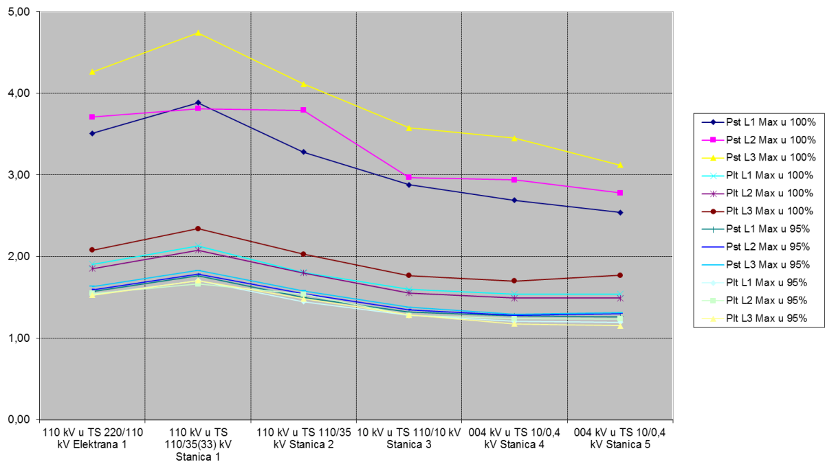
Slika 6.4. Usporedba vrijednosti flikera po mjernim točkama, P_{st} i P_{lt} u 100% i 95% vremena po fazama i po mjernim točkama
