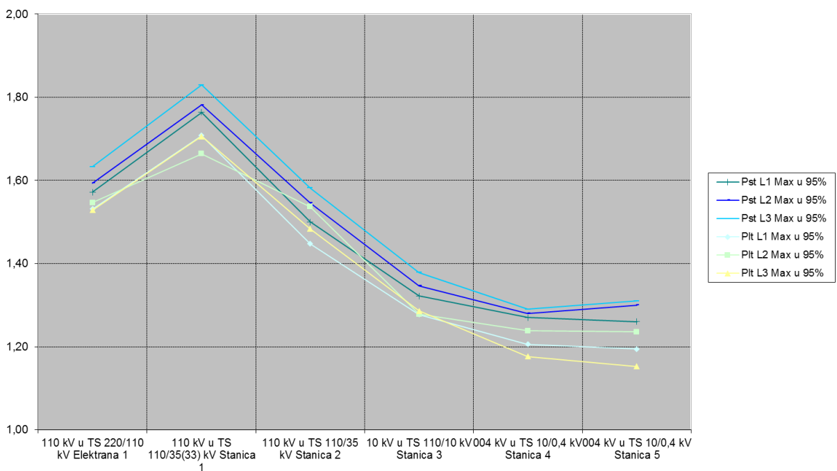
Slika 6.3. Usporedba vrijednosti flikera po mjernim točkama, P_{st} i P_{lt} u 95% vremena po fazama i po mjernim točkama
