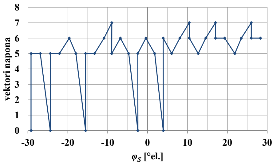
Slika 9.7. Simulacijski rezultati, prediktivno upravljanje momentom ( n = n_n , m_{elmAV} = M_n , \psi_{sref} = |\psi_{sn}| , u_{dc} = 600 V, \Delta T = 80 \mu s, \lambda = 4 Nm/mVs): primijenjeni vektori napona izmjenjivača u četvrtom sektoru
