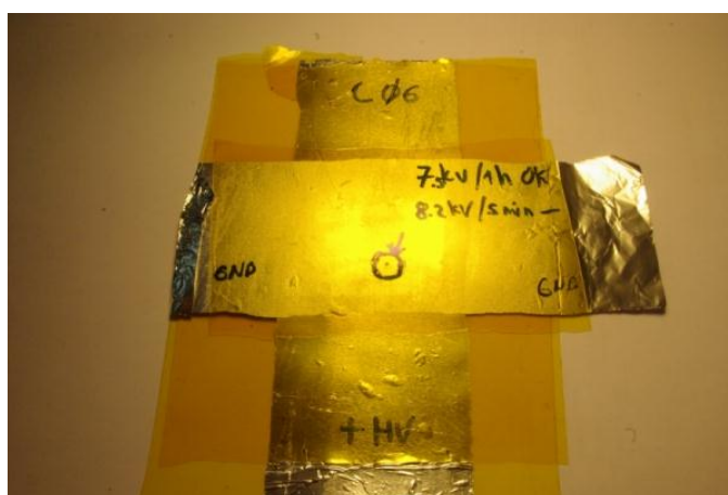
Slika 6.34. Pločasti kondenzator nakon ispitivanja probojnog napona. Strelica s krugom označava mjesto proboja. Elektrode su napravljene od aluminijske folije za kućanstvo. Na ovoj slici je testiran Kapton debljine 0,1 milimetar koji ima adhezivni sloj s obje strane.
