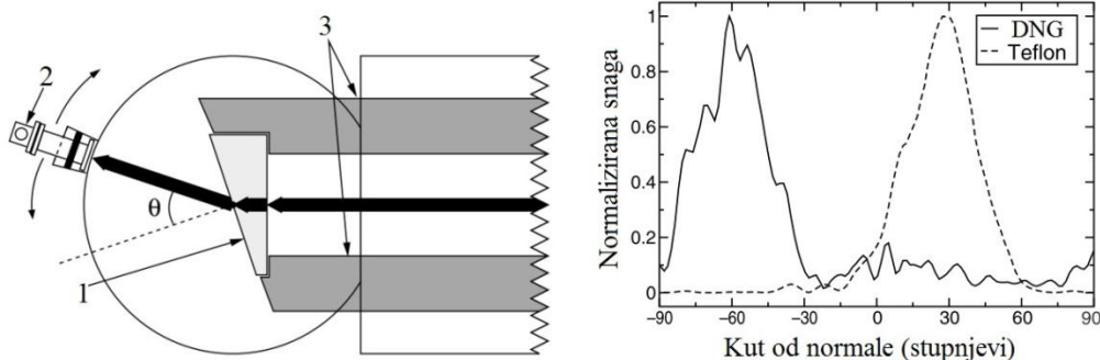
Slika 2.15 - Lijevo: mjerni postav eksperimenta sastojao se od prizme (1) s kutom 18.4 stupnja prema incidentnoj zruci načinjene od teflona ili DNG metamaterija smještene između dva diska od aluminija, detektora mikrovalne energije (2) koji je smješten na goniometru s rezolucijom mjerenja od 1.5 stupnja te od mikrovalnog apsorbera (3). Crne strelice označavaju smjer kretanja mikrovalne energije prilikom mjerenja prizme od teflona. Desno: Prenesena snaga na 10.5 GHz kao funkcija kuta refrakcije za teflon (puna linija) i za DNG metamaterijal (isprekidana linija). Izračunati indeks loma za DNG materijal iznosi -2.7. Preuzeto iz [4].
