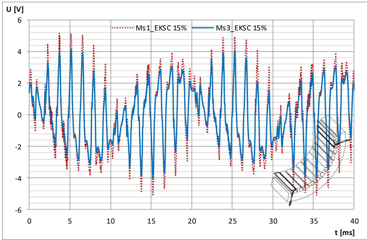
Slika 5.12 Usporedba valnih oblika induciranog napona u mjernim svicima Ms1 i Ms3 prostorno razmaknutih za 2\tau_p kod iznosa statičkog ekscentriciteta od 15 % zračnog raspora (pomak u smjeru + y osi)
