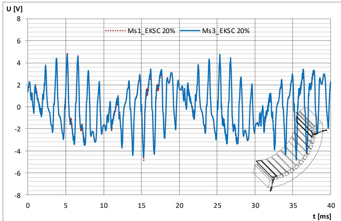
Slika 5.36 Usporedba valnih oblika inducirano napona u mjernim svicima Ms1 i Ms3 prostorno razmaknutih za 2\tau_p kod iznosa statičkog ekscentriciteta od 20 % zračnog raspora (pomak u smjeru + x osi)
