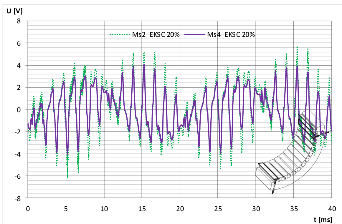
Slika 5.35 Usporedba valnih oblika inducirano napona u mjernim svicima Ms2 i Ms4 prostorno razmaknutih za 2\tau_p kod iznosa statičkog ekscentriciteta od 20 % zračnog raspora (pomak u smjeru + x osi)
