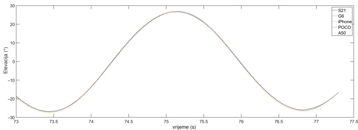
Slika 3.23: Elevacija izračunata za jedan titraj njihala za svih pet pametnih telefona.
