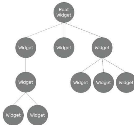
Slika 22. Stablo widgeta [1]
