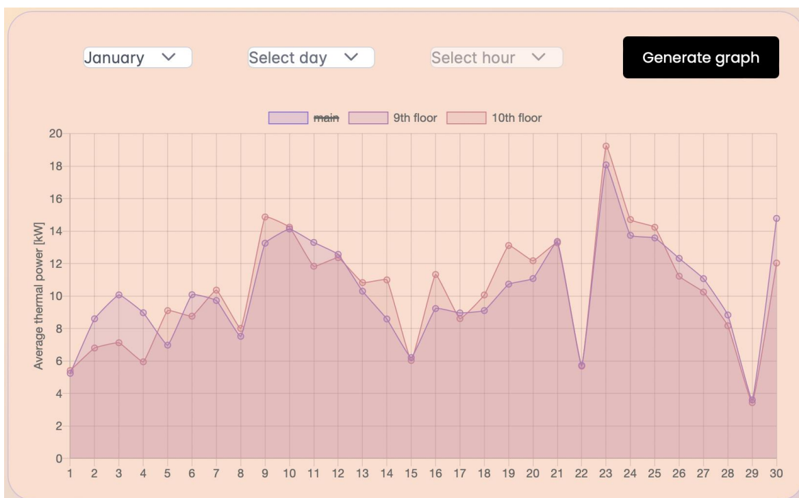
Slika 3.5 Grafikon povijesnih podataka 9. i 10. kata za 1. mjesec 2022. godine.
