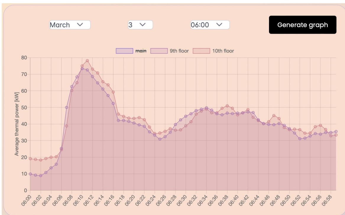
Slika 3.11 Grafikon povijesnih podataka 9. i 10. kata za 3.3.2022. od 06:00 do 06:59 sati.
