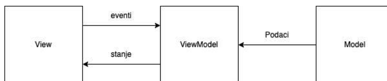
Slika 15 Graf MVVM arhitekture
