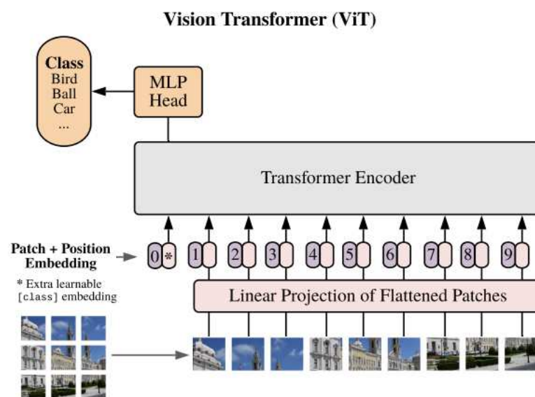
Slika 2. Arhitektura Vision Transformer a kao ulaz prihvaća sliku te ju dijeli na okna koja se pretvaraju u vektore. Tim vektorima se također ugradi i informacija o poziciji [1]. Vektorima iz slike se također dodaje i učeni [CLS] vektor te svi ti vektori prolaze kroz sliku i međusobno djeluju jedno na drugo. Na kraju pomoću klasifikacijske glave se slika može klasificirati. [4]
