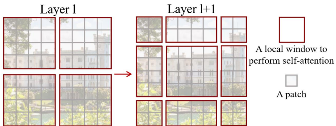
Slika 3. Prikaz slojeva u Swin Transformeru . Počinjemo sa podjelom slike po okvirima. Te okvire možemo gledati kao sliku koja ulazi u ViT . Ti okviri su podijeljeni u dodatna kvadratna okna koja čine ulaze u sloj pažnje te samo elementi u istom okviru se međusobno vide. U idućim slojevima se mijenjanju pozicije i veličine okvira te novi elementi iz slike vide druge nove elemente. [5]
