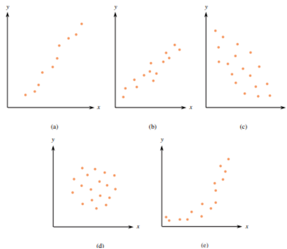
Slika 4.6 Prikaz korelacije između dvije varijable Izvor: Introduction to Statistics and Data Analysis, stranica:300 [20]
