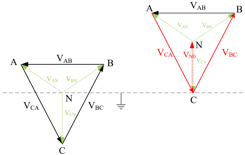
Slika 2.4: Fazorski dijagram napona pri metalnom zemljospoju
