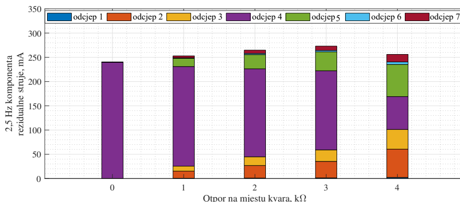
Slika 5.11: 2,5 Hz komponenta u rezidualnim strujama po odcjepima ovisno o otporu na mjestu kvara, za slučaj kvara 2 (kraju odcjeka 4)
