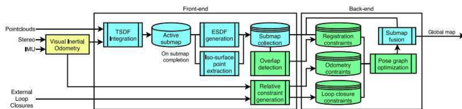
Slika 3.6: Voxgraph pregled [3]
