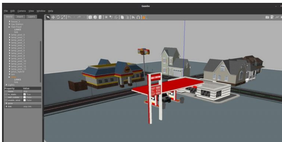
Slika 2.3: Gazebo simulator [15]
