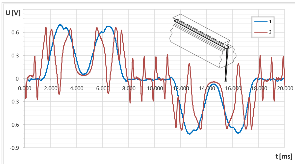
Slika 8.5. Napon induciran u mjernom svitku Ms_1 , za prazni hod: Krivulja 1 – mjerenje, Krivulja 2 – izračun.
