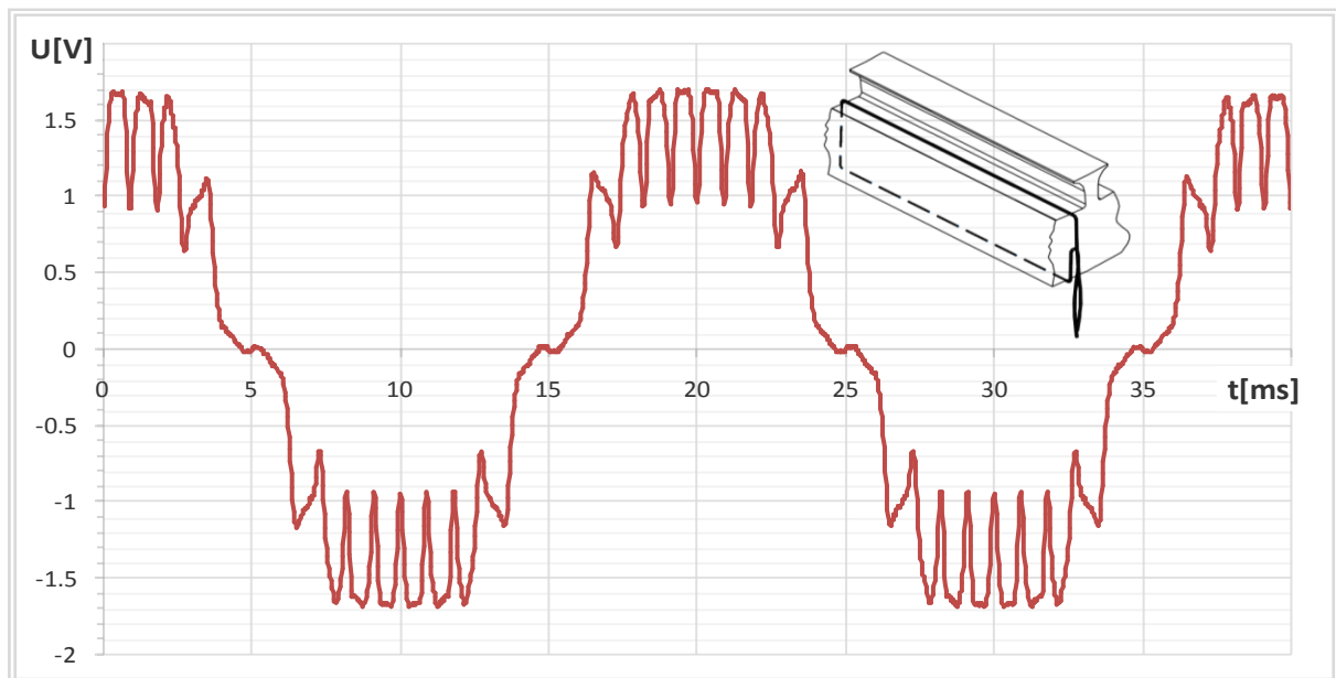
Slika 6.50. Napon induciran u mjernom svitku Ms_3 i Ms_4 , za prazni hod pri uzbuđnoj struji od 8,7 A, uz smanjeni iznos broja zavoja jednog pola za 10 %.
