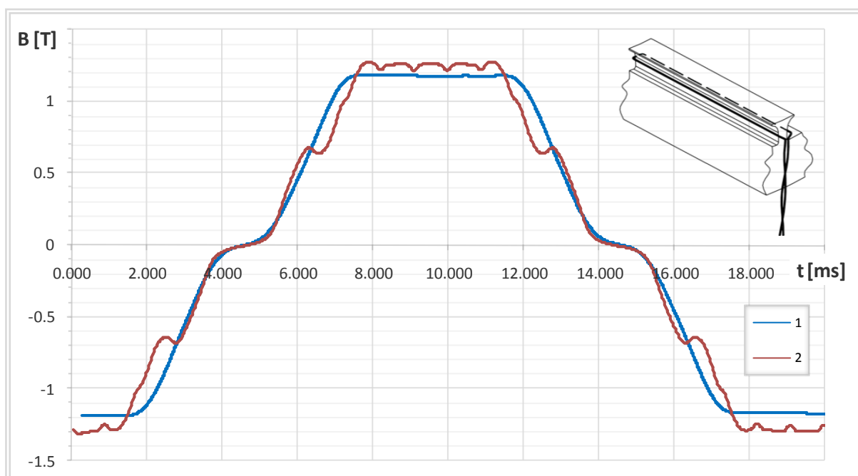
Slika 8.6. Raspodjela magnetske indukcije dobivena integracijom napona induciranog u mjernom svitku Ms_1 , za prazni hod: Krivulja 1 – mjerenje, Krivulja 2 – izračun.
