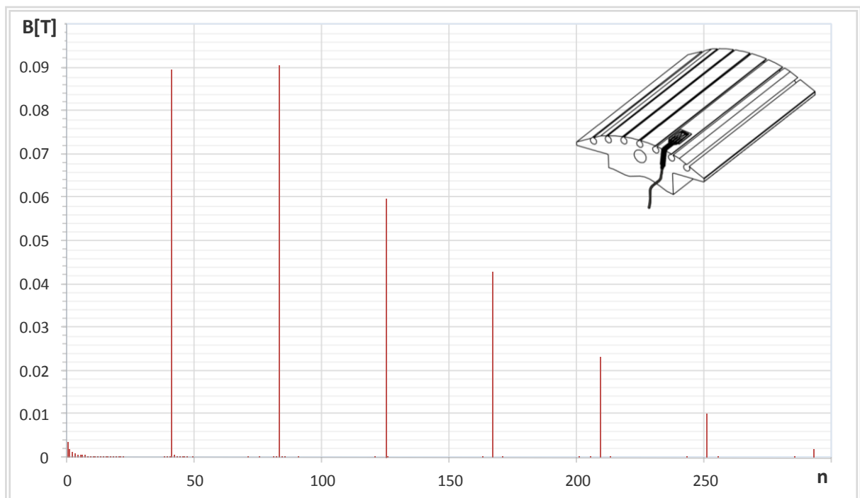
Slika 6.77. Frekvencijska analiza raspodjele magnetske indukcije u zračnom rasporu promatrana s polne papučice generatora u praznom hodu, bez prisutnosti kratkih spojeva zavoja svitka namota armature.
