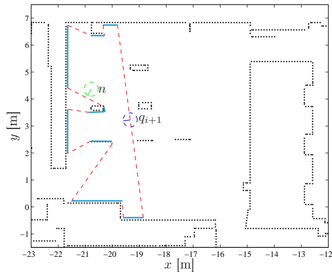
Slika 4.20. Određivanje skočnih bridova (crtkane linije) i linijskih segmenta (pune linije) iz odabranog sljedećeg mjernog položaja q_{i+1} .
