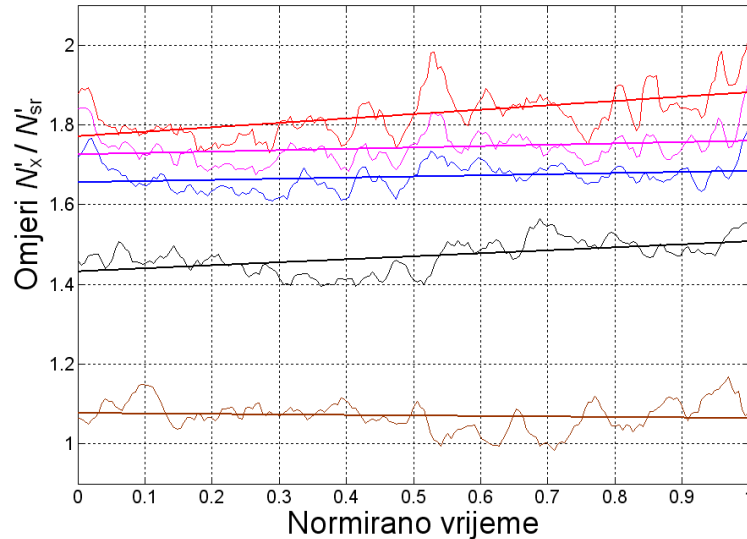
Slika 2.37. Promjena omjera parametara N'_1 , N'_5 , N'_{10} , N'_{25} i N'_{50} i srednje vrijednosti specifične glasnoće N'_{sr} u ovisnosti o vremenu
