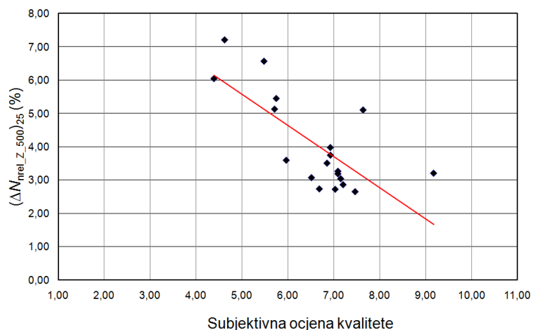
Slika 5.11. Raspršni grafikon subjektivnih ocjena kvalitete za zvuk uređaja pri zaustavljanju u odnosu na postotni percentil kolebanja glasnoće (\Delta N_{\text{rel}_Z_{500}})_{25}
