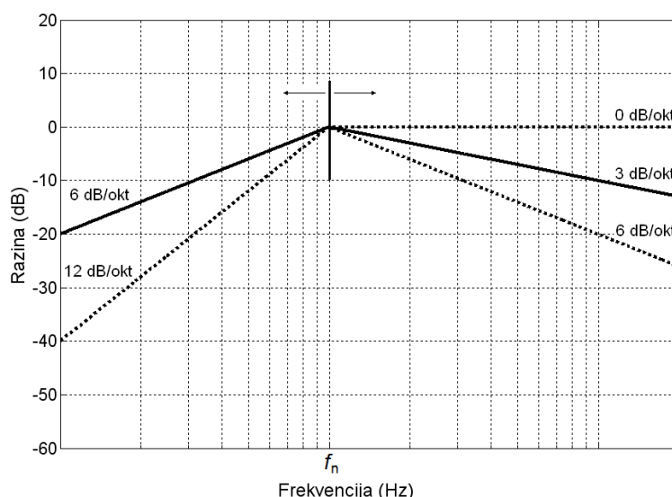
Slika 3.9. Oblikovanje širokopojasnog šuma
