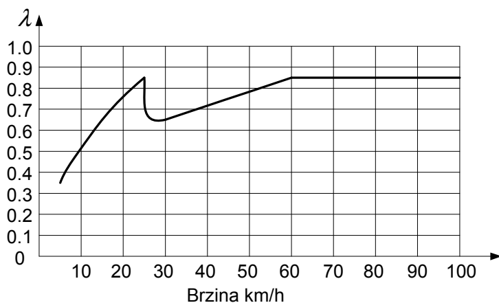
Slika 3.3. Krivulja faktora snage \lambda elektromotornoga vlaka
