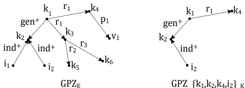
Slika 4.10. Primjer konceptne restrikcije grafa područnog znanja
