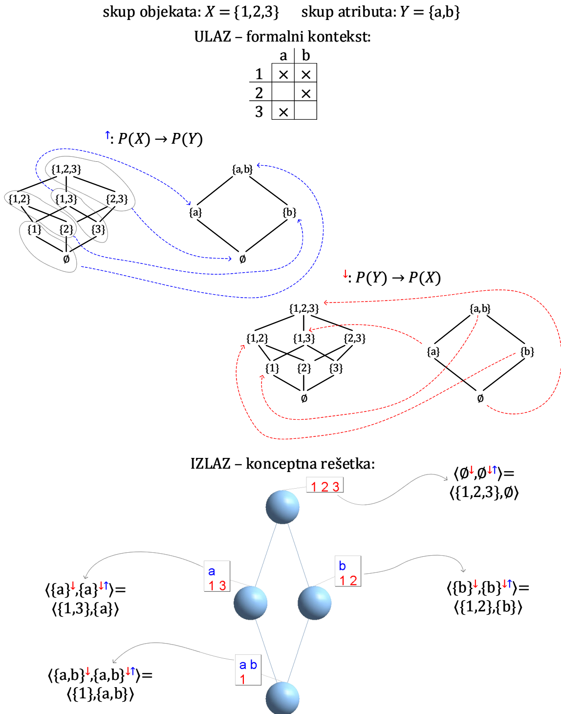
Slika 3.8: Prikaz provođenja metode FCA
