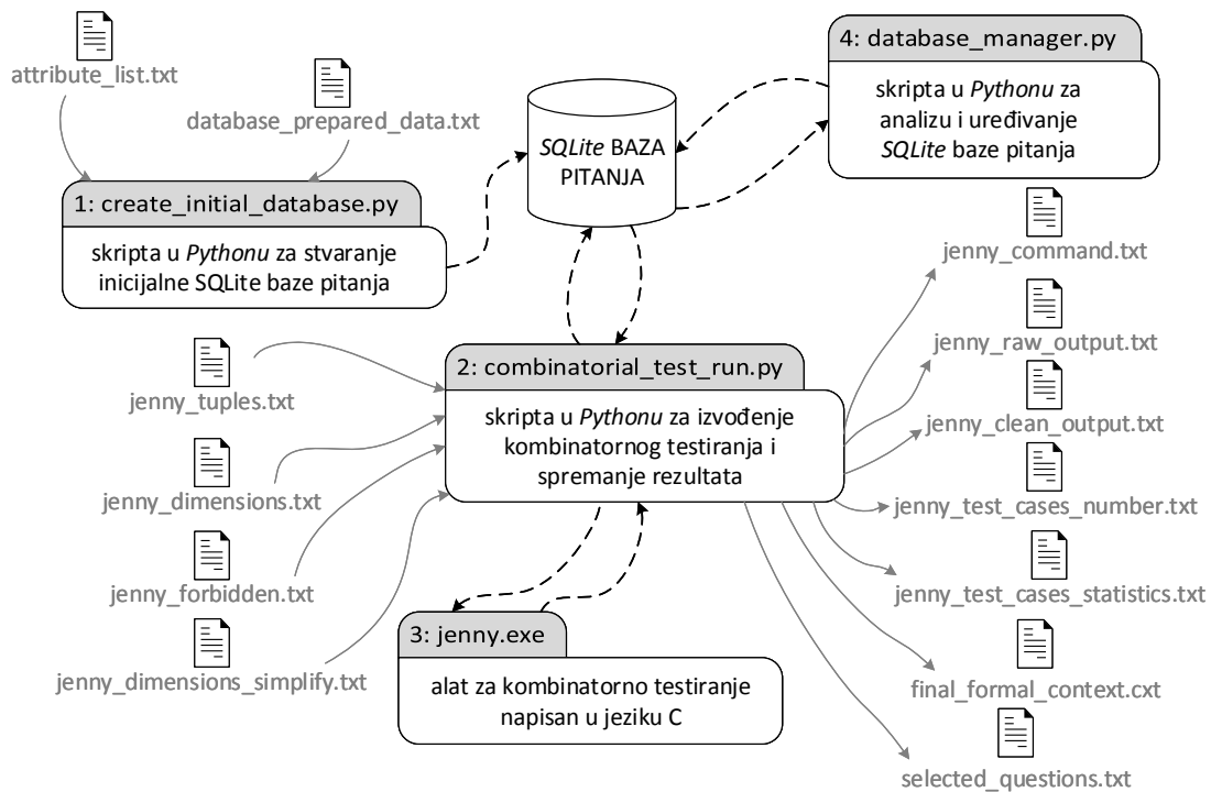
Slika 5.2: Pregled modula za kombinatorno testiranje
