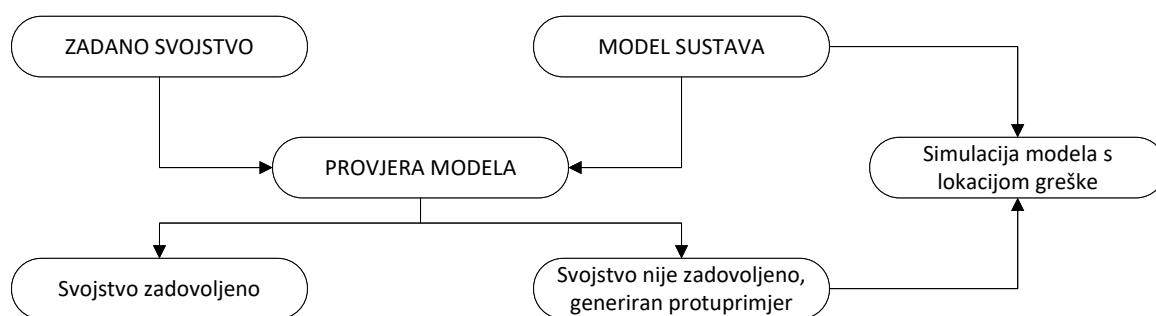
Slika 3.29: Opis procesa provjere modela
