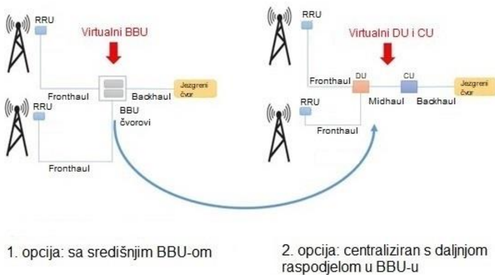
Slika 2.8 vRAN [10]
