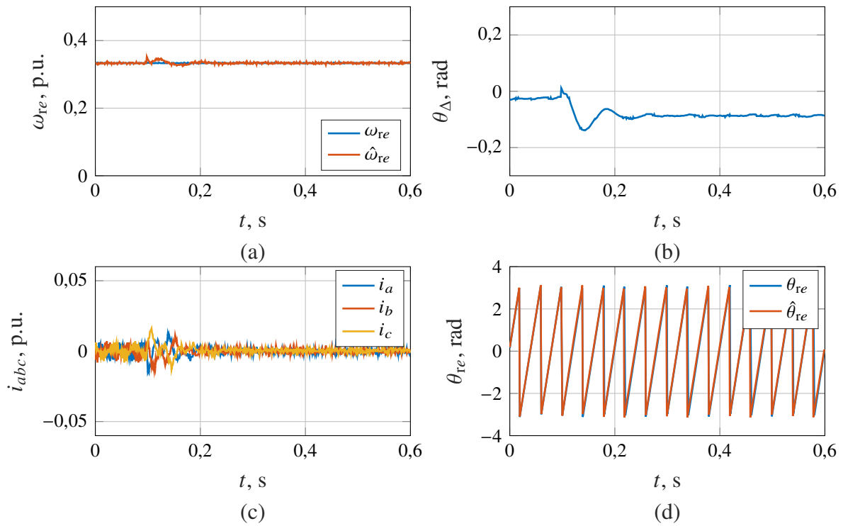
Slika 8.15. Uklop IPM-a pri brzini vrtnje \omega_{re} = 0,33 p.u. s kompenzacijom kašnjenja digitalnog sustava. (a) Mjerena i estimirana vrijednost brzine vrtnje. (b) Greška kuta. (c) Mjerene struje. (d) Mjereni i estimirani kut.
