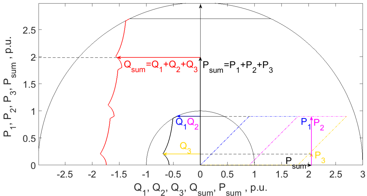
Slika 6.3: Određivanje granica u kapacitivnom dijelu zajedničke pogonske karte grupe jednakih generatora u sekvencijalnom terećenju
