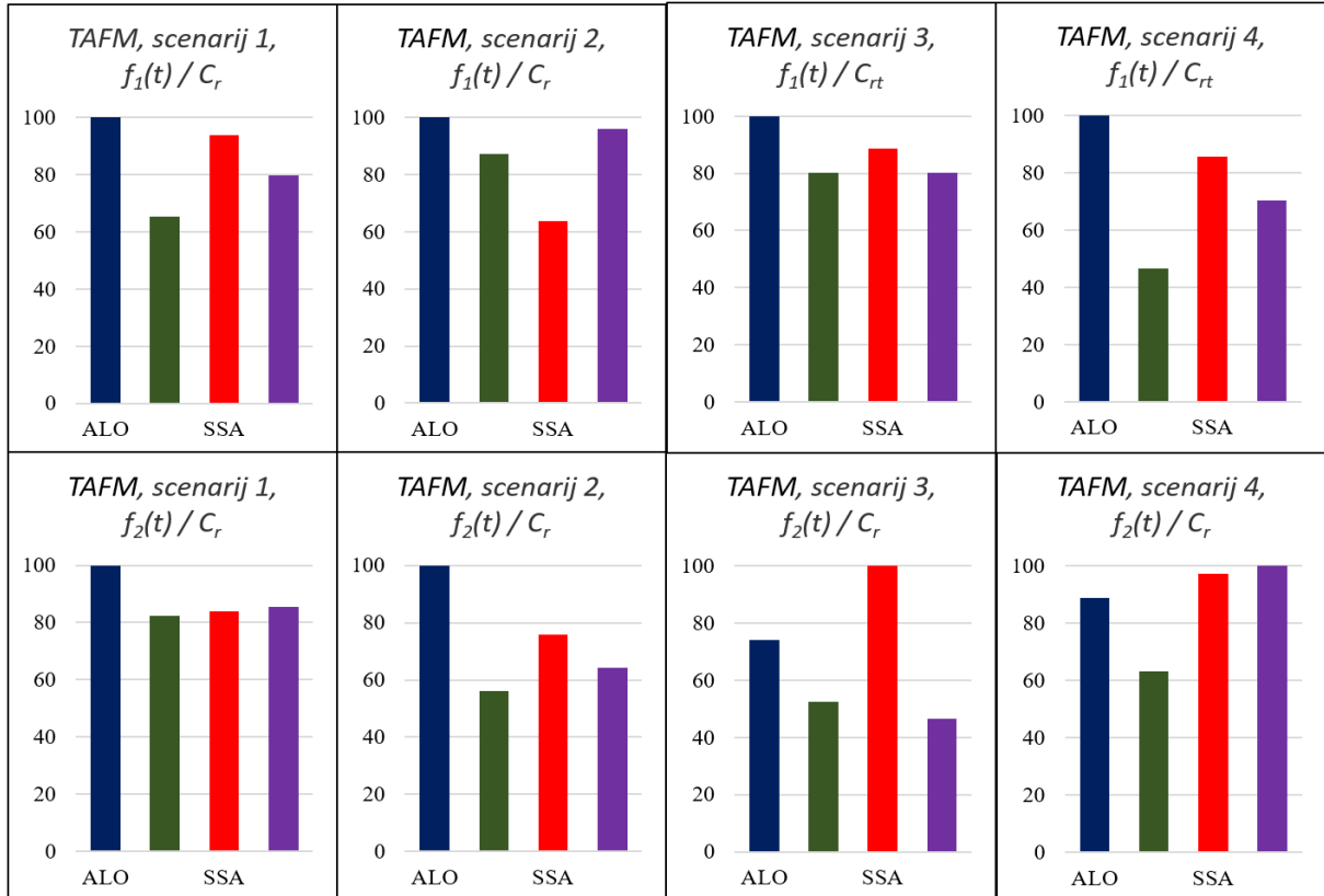
Slika 6.61. TAFM – pregled moći konvergencije C_r algoritama po scenarijima i metodama
