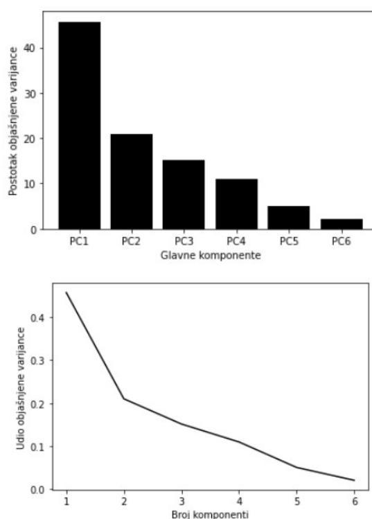
Slika 38. Prikaz postotka objašnjene varijance pomoću glavnih komponenta benchmarka na periodu COVID 19 pandemije
