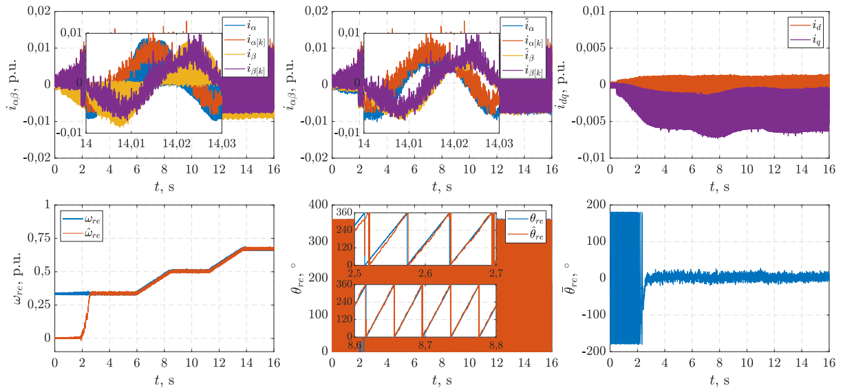
(a) Estimacija kuta i brzine vrtnje pri isprekidanom radu pretvarača i promjeni brzine vrtnje
