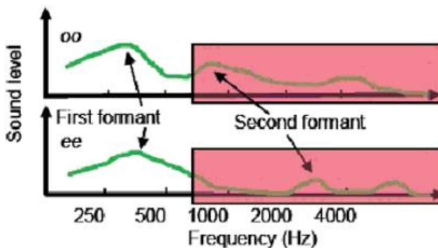
Slika 1.12: Položaj F1 i F2 kod glasova „o“ i „e“ [5]
