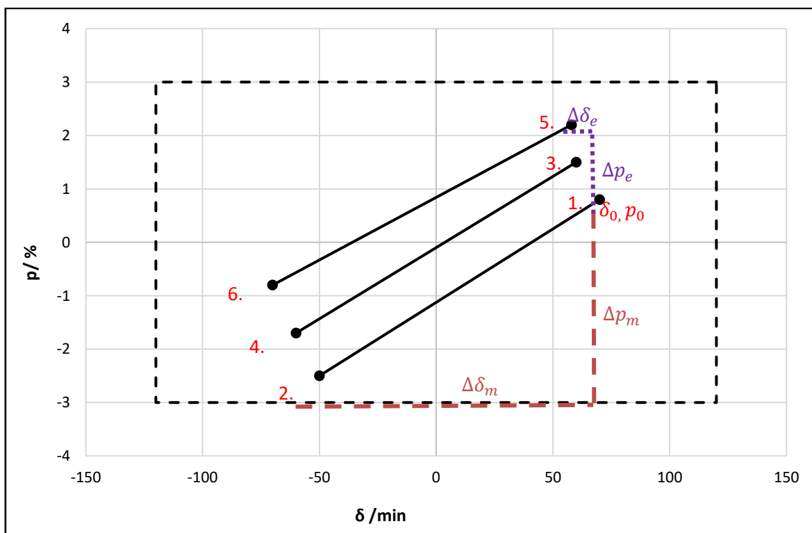
Slika 44. Ispitne točke za dokazivanje klase točnosti na mjernom namotu
