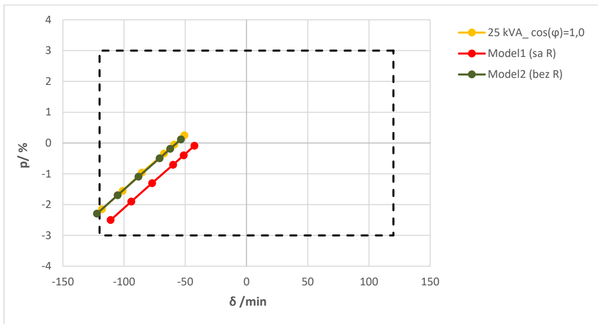
Slika 36. Rezultati ispitivanja uz korekcijski sklop s manjim induktivitetom za 25 kVA \cos\phi=1,0
