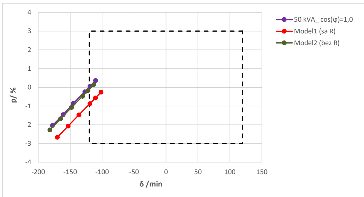
Slika 37. Usporedba rezultati ispitivanja i numeričkih modela uz korekcijski sklop s manjim induktivitetom za 50 kVA \cos\phi=1,0
