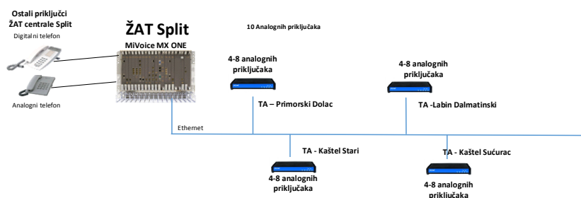
Slika 8.12. ŽAT-C Split-prikaz postojećeg i novog stanja udaljenih korisnika
