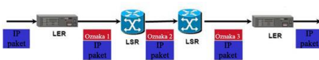
Slika 7.3. Prikaz prolaska paketa kroz LSP [11]
