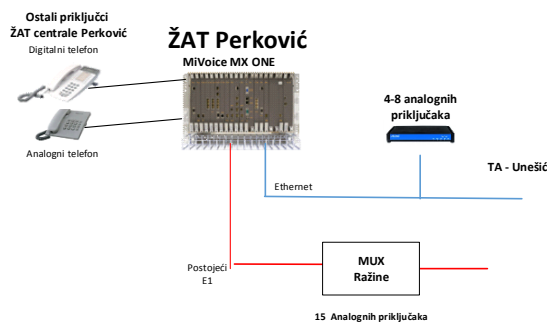
Slika 8.11. ŽAT-C Perković-prikaz postojećeg i novog stanja udaljenih korisnika
