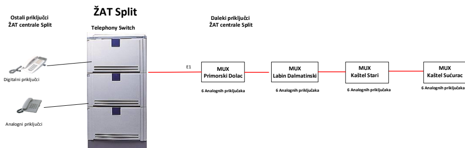
Postojeće stanje ŽAT sustava Split
