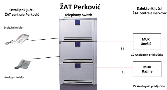
Prijedlog novog stanja ŽAT sustava Perković
