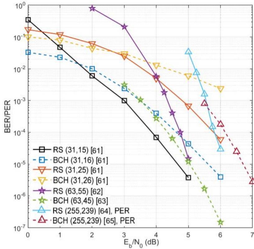
SI.2.15 Usporedba BCH i RS koda za različite omjere kodova [21]
