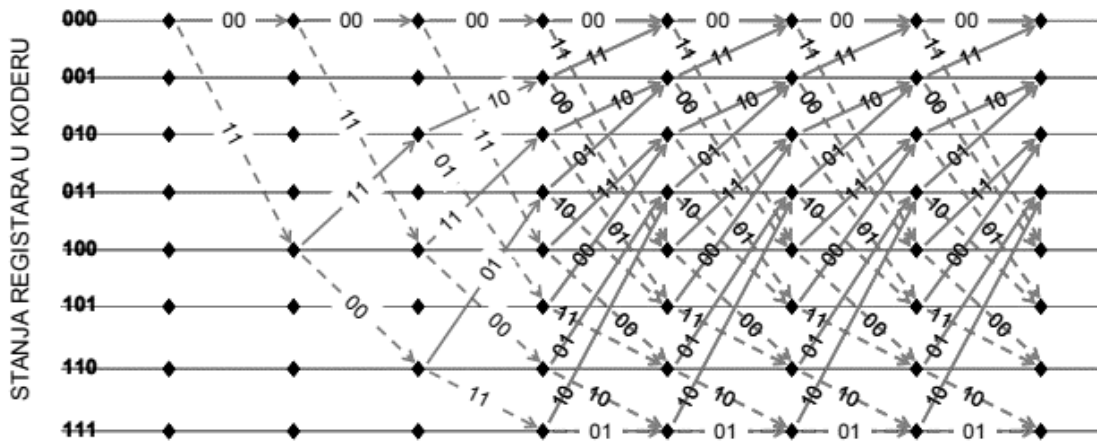
Sl.2.6 Dijagram rešetke za (2,1,4) kod
