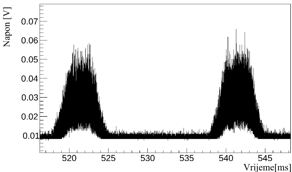
Slika 5.16: Dio izvornog signala na izlazu SiPM detektora uzrokovan detekcijom dva impulsa rendgenskog zračenja.
