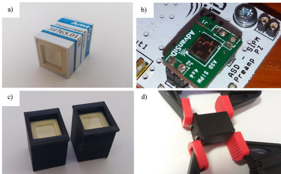
Slika 5.6: a) NaI(Tl) kristal smješten u hermetički zatvoreno kućište, b) SiPM na koji je nanescena optička spojna mast, zalemljen je na elektroničku pločicu, c) dva kristala smještena u kućište detektora d) sastavljeni detektor.
