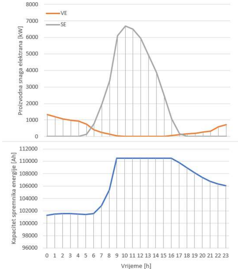
Slika 2.17: primjer dinamike proizvodnje energije iz VE i SE i utjecaj na dinamiku kapaciteta spremnika energije
