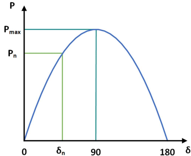
Slika 2.5. Krivulja opterećenja
