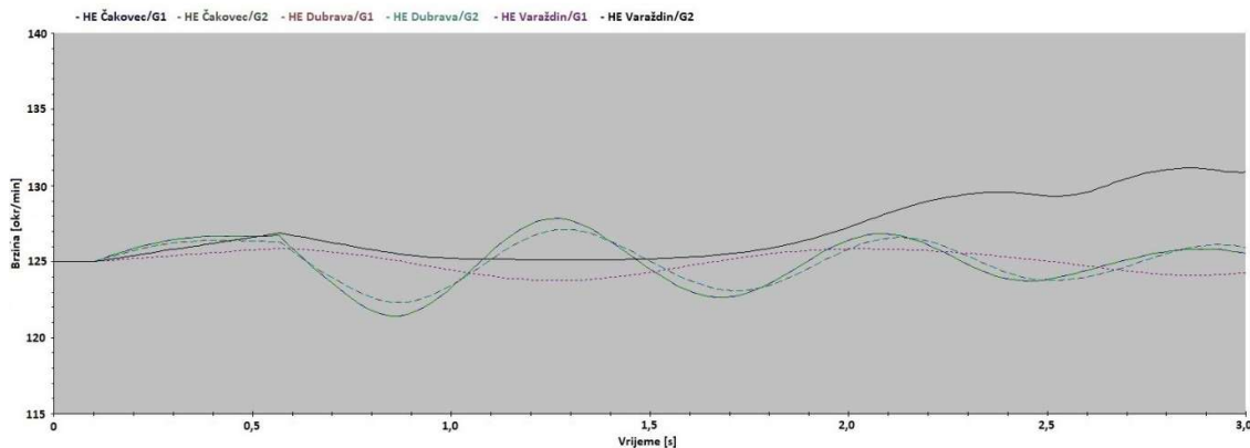
Slika 4.21. Rezultati simulacija za brzinu vrtnje generatora 2 za vrijeme troleznog kratkog spoja na sabirnicama HE Varaždin s trajanjem kvara od 468 ms
