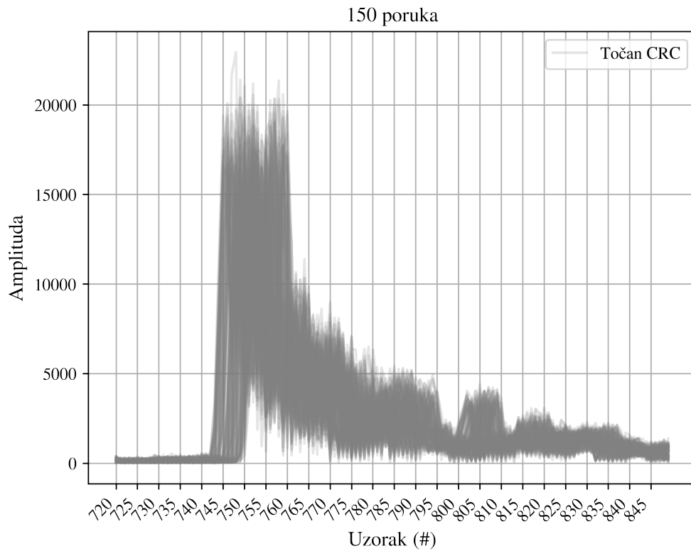
Slika 4.21: CIR bez generiranih smetnji (izmjereno u prostoriji na fakultetu)
