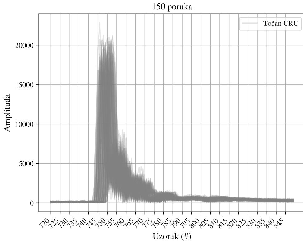
Slika 4.17: CIR uz IEEE 802.11b komunikaciju (izmjereno u EMC komori)
