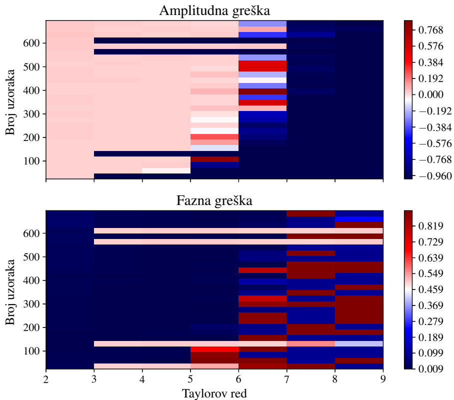
(a) Prikaz pogreške s obzirom na broj uzoraka i stupanj Taylorovog reda
