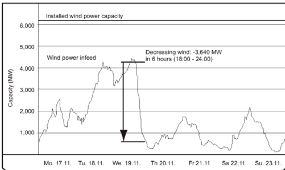
Slika 1.30 Fluktucija snage ukupne proizvodnje svih vjetroelektrana u prijenosnom sustavu mreže operatora E.ON Netz u Njemačkoj 2007.
