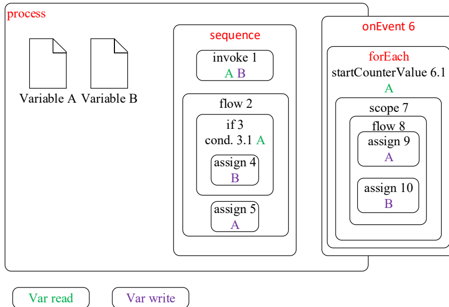
Slika 50: BPEL proces iz tablice 12
