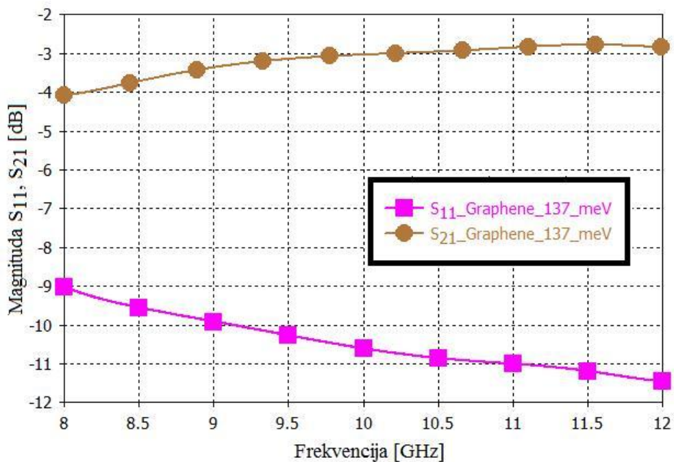
Slika 6.8. Moduli raspršnih parametara S_{11} i S_{21} dobiveni simulacijom jednoslojnog grafena polariziranog naponom 2,5 kV ( \mu_c=137 meV) ili dvoslojnog nepolariziranog grafena ukupnog površinskog otpora 615 \Omega/\square . Debljina 3D materijala je 0,2 mm a vodljivost mu je 7,97 S/m.
