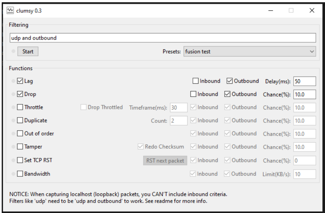
Slika 5.3 Primjer konfiguracije u programu Clumsy
