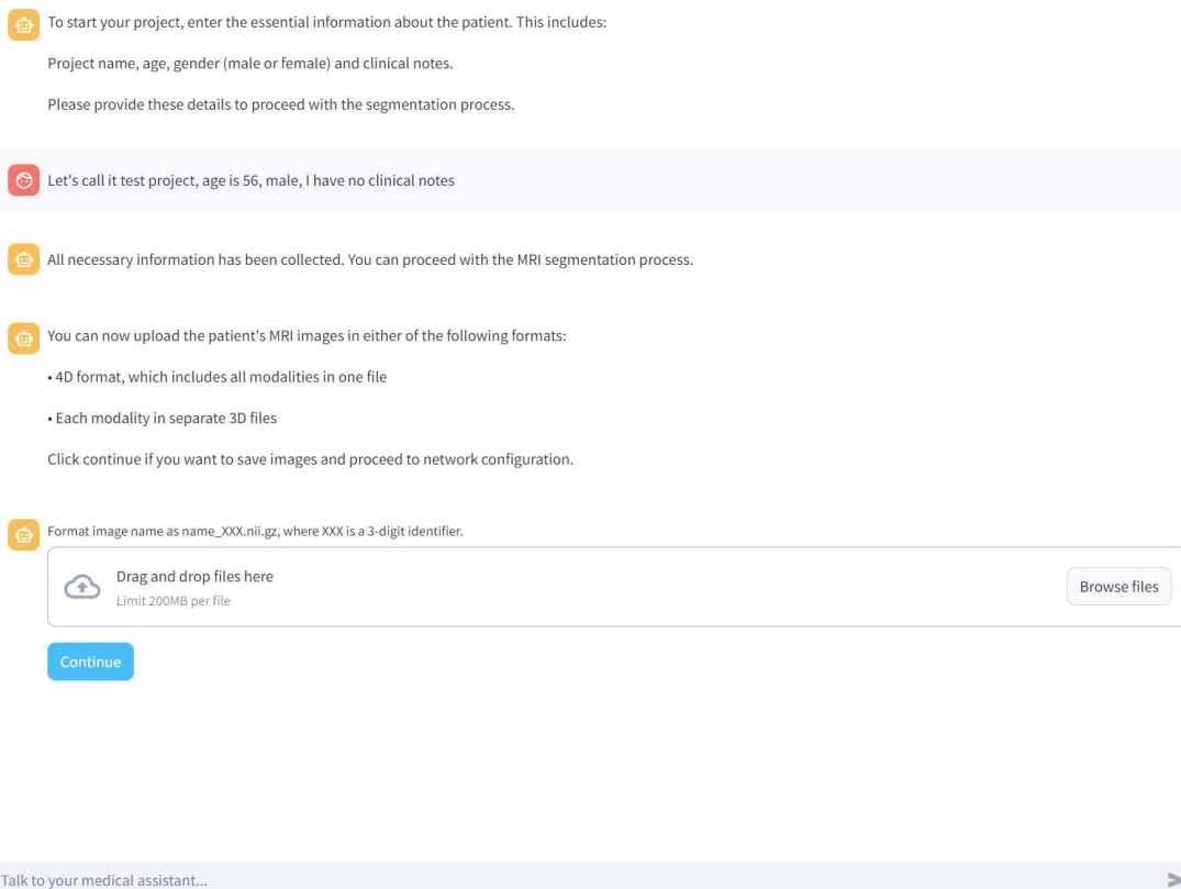
Slika 6.1. Inicijalizacija projekta
