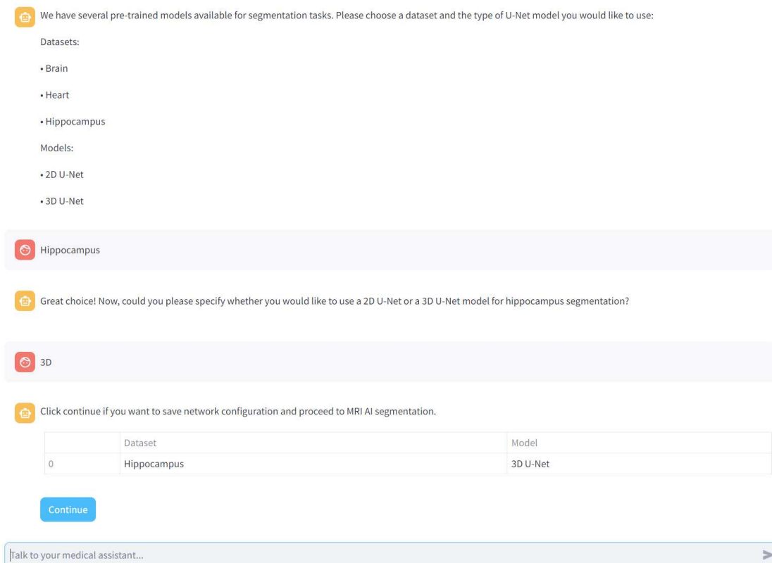
Slika 6.2. Odabir skupa podataka i arhitekture mreže
